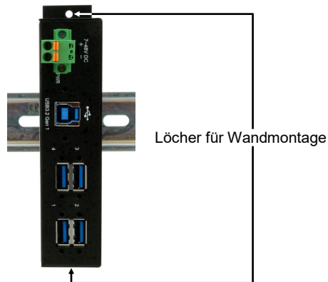
Montage an Tragschiene
